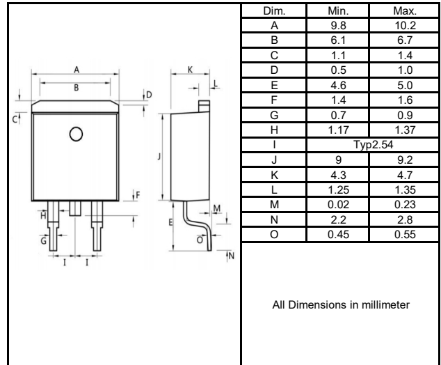
TO-263C
